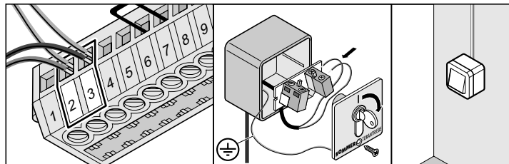
Контакты 2 + 3 подключение выключателя 1
