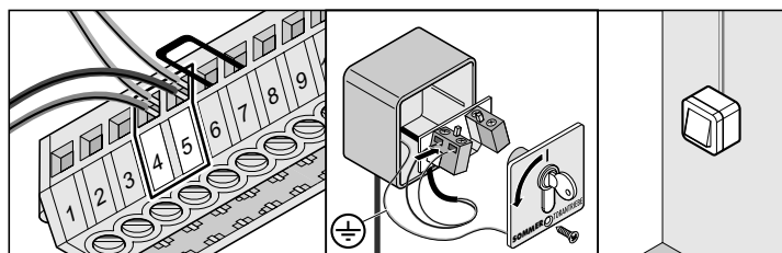
Контакты 4 + 5 подключение выключателя 2
